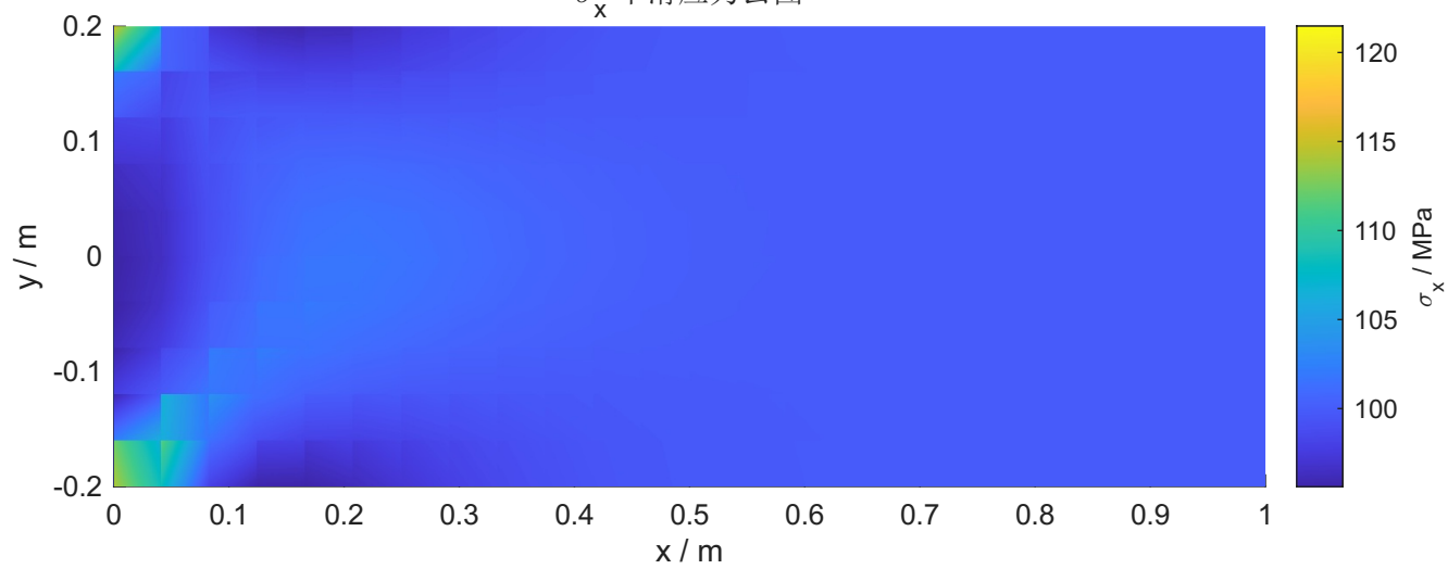
\sigma_x 平滑应力云图
